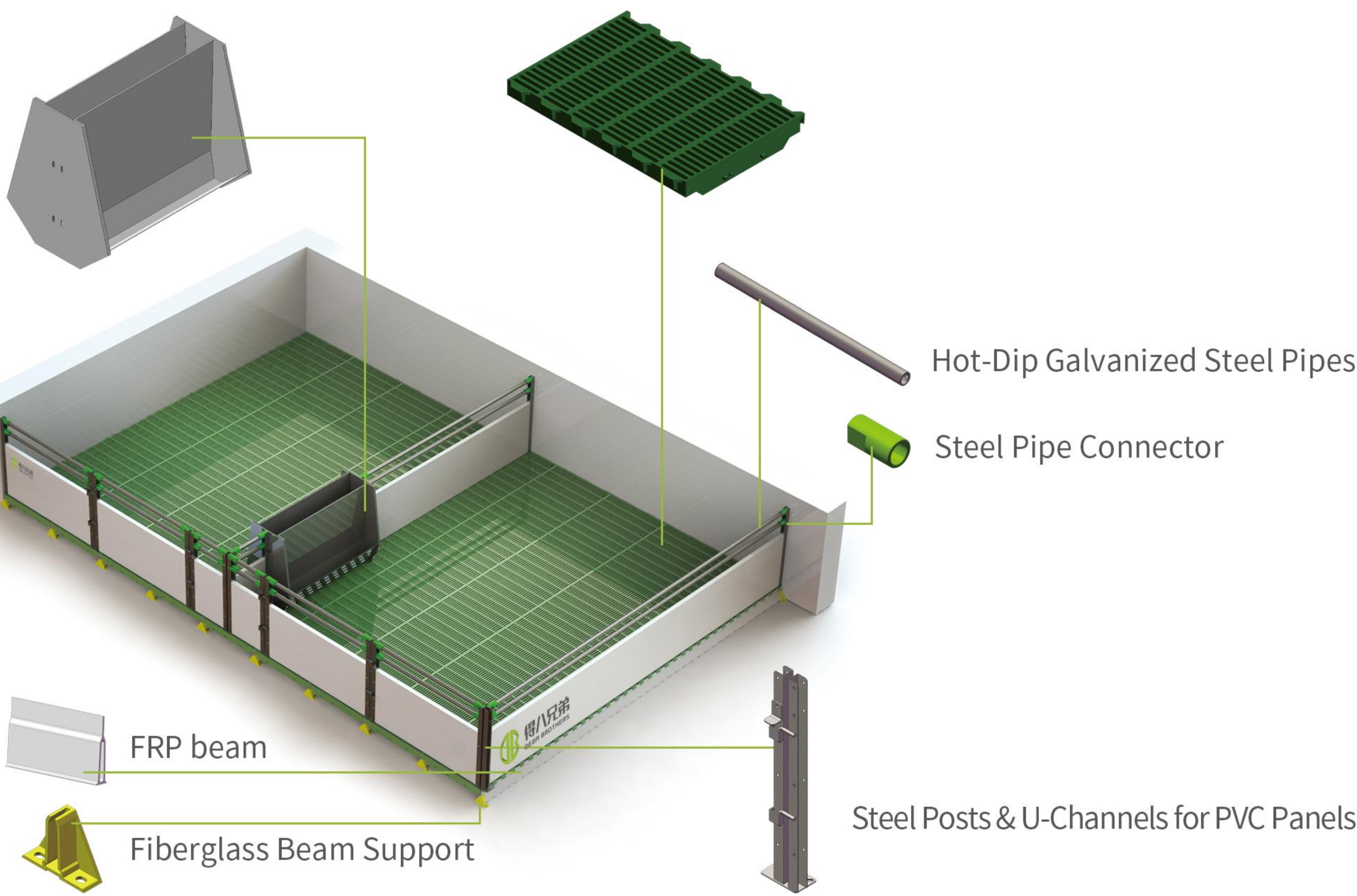
Interlocking Plastic Slats
